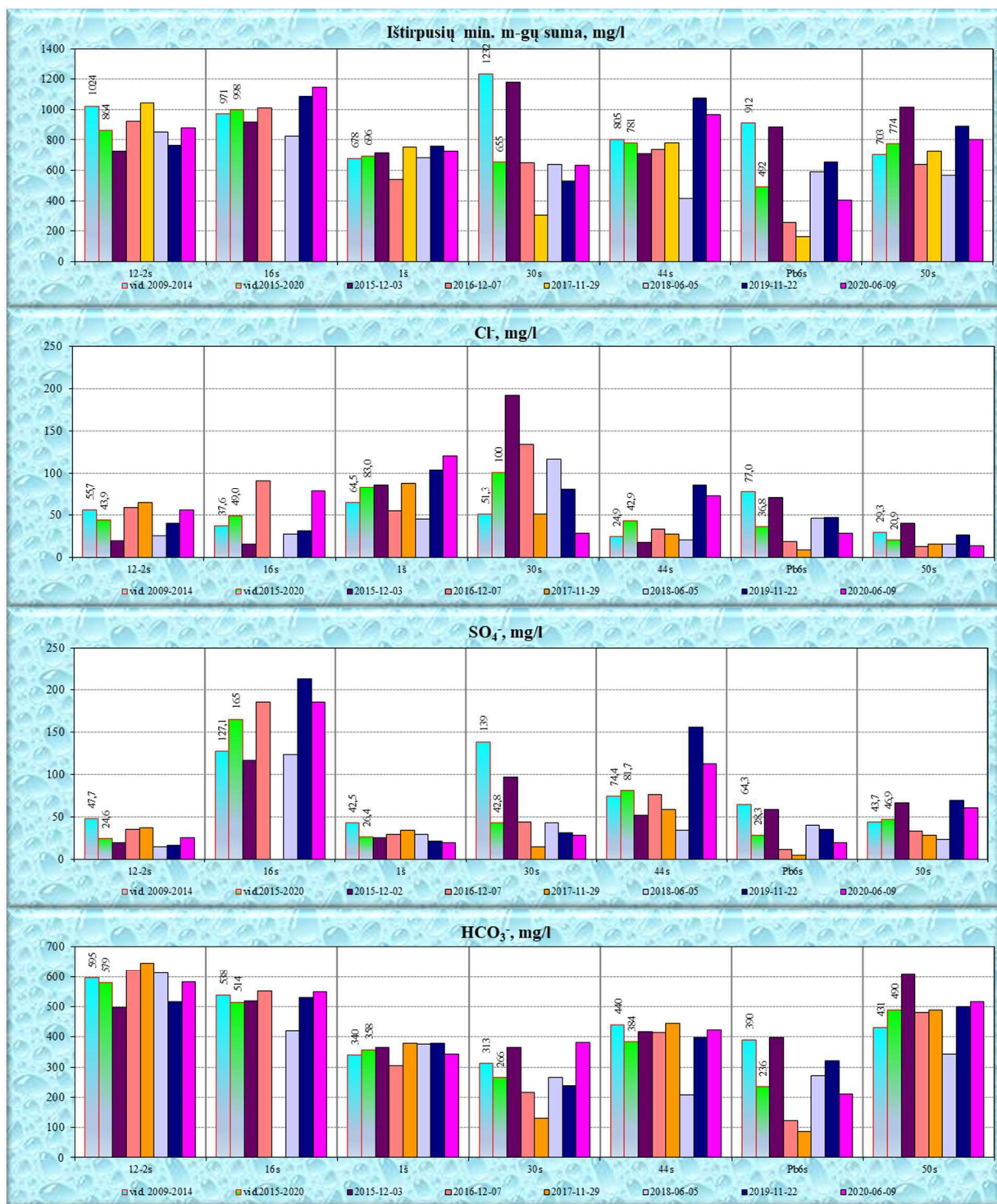
32 pav. Šulinių gruntinio vandens cheminės sudėties pokyčiai 2015–2020 m. ir vidutinės koncentracijos 2009–2014 m. (BIMMS, pagrindiniai anijonai)
