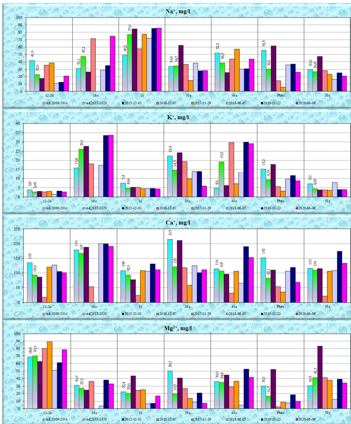
33 pav. Šiaulių gruntinio vandens cheminės sudėties pokyčiai 2015–2020 m. ir vidutinės koncentracijos 2009–2014 m. (pagrindiniai kationai)
