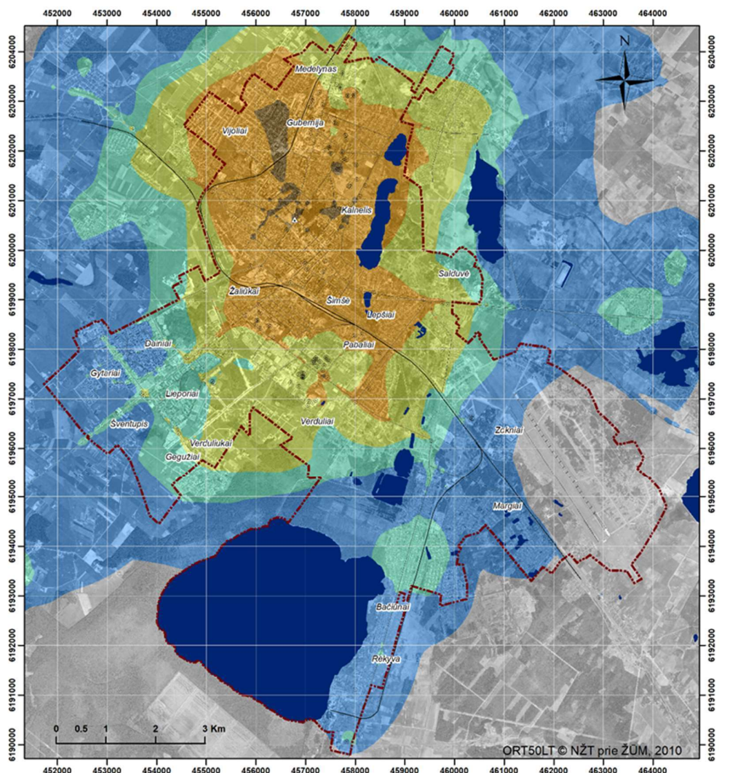
Vidutinė metinė kietųjų dalelių ( KD_{10} ) koncentracija ( \mu\text{g}/\text{m}^3 ) aplinkos ore Šiauliuose 2019 m.
