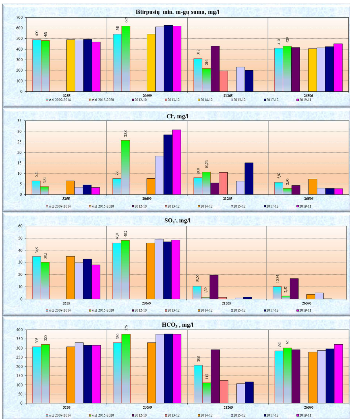
42 pav. Gręžinių viršutinio permo požeminio vandens cheminės sudėties pokyčiai 2012–2020 m. ir vidutinės koncentracijos (BIMMS, pagrindiniai anijonai)
