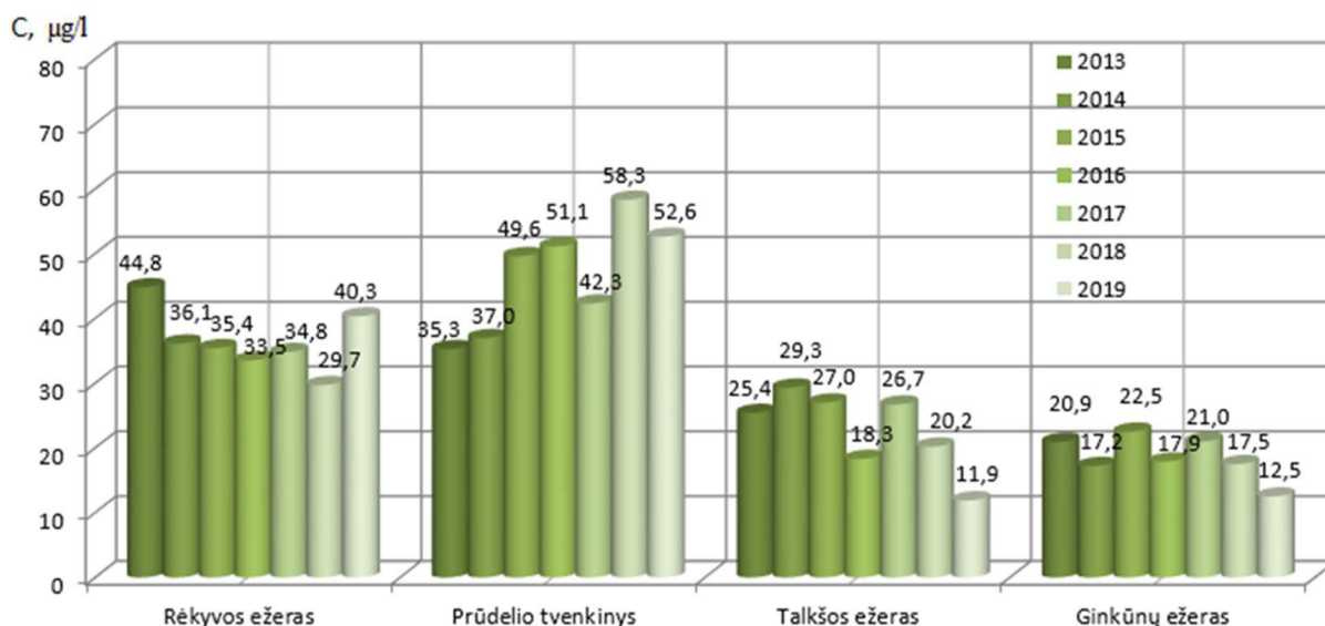
16 pav. Vidutinės metų chlorofilo „a“ koncentracijos kitimas Šiaulių miesto paviršiniuose vandens telkiniuose 2013–2019 m.
