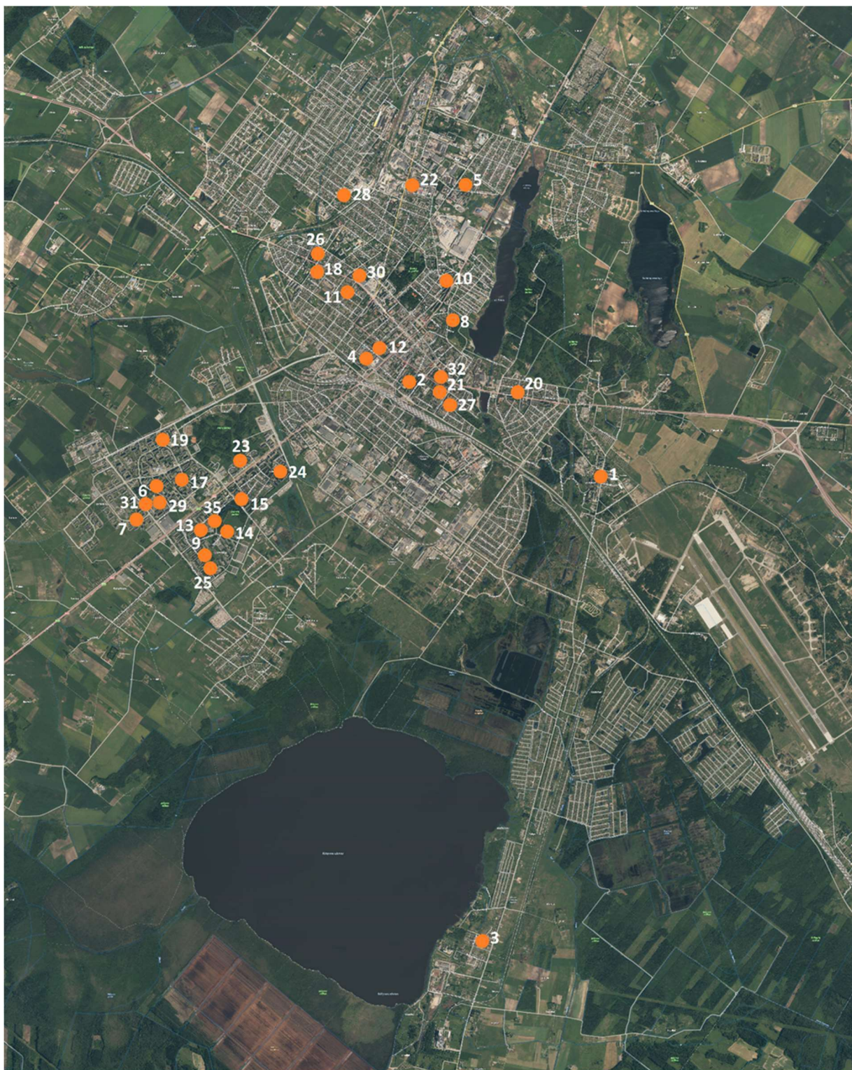
19 pav. Triukšmo matavimo vietos Šiauliuose (lopšelių-darželių aplinkoje)
