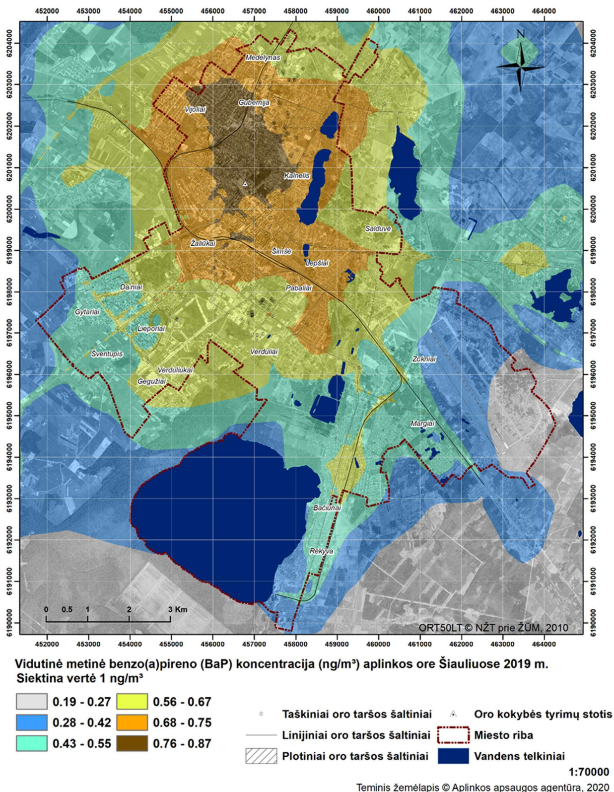
10 pav. Vidutinė metinė benzo(a)pireno (BaP) koncentracija Šiaulių m. aplinkos ore 2019 m.
