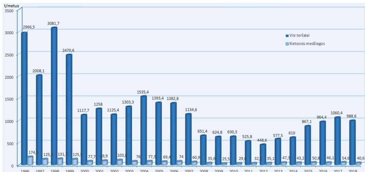
2 pav. Stacionarių aplinkos oro taršos šaltinių emisijų kiekio kitimas Šiauliuose 1996–2018 m. laikotarpiu.
