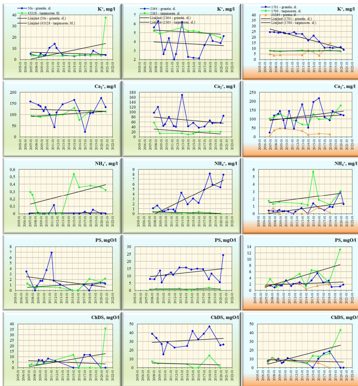
46 pav. Gruntinio, tarpmoreninio ir permo sluoksnių požeminio vandens cheminės sudėties rodiklių kaitos grafikai (tęsinys)
