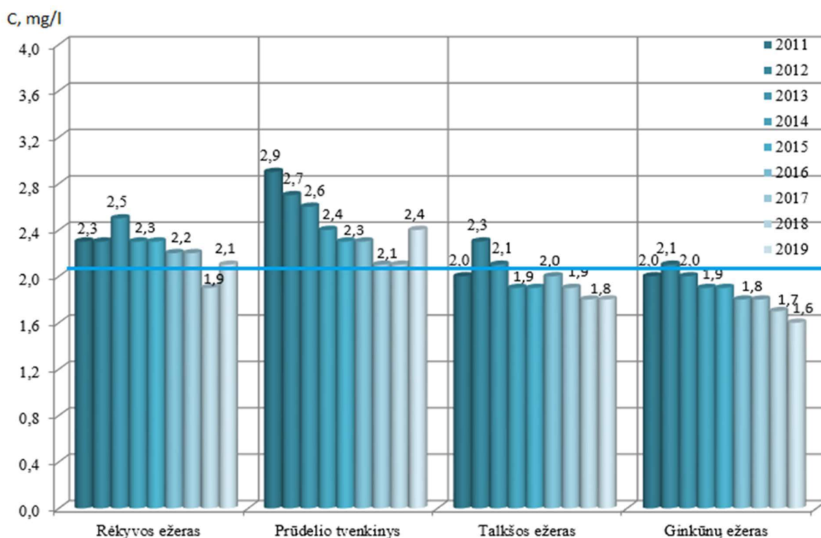
14 pav. Bendrojo azoto ( N_b ) vidutinės metų koncentracijos kitimas paviršiniuose vandens telkiniuose 2011–2019 m.
