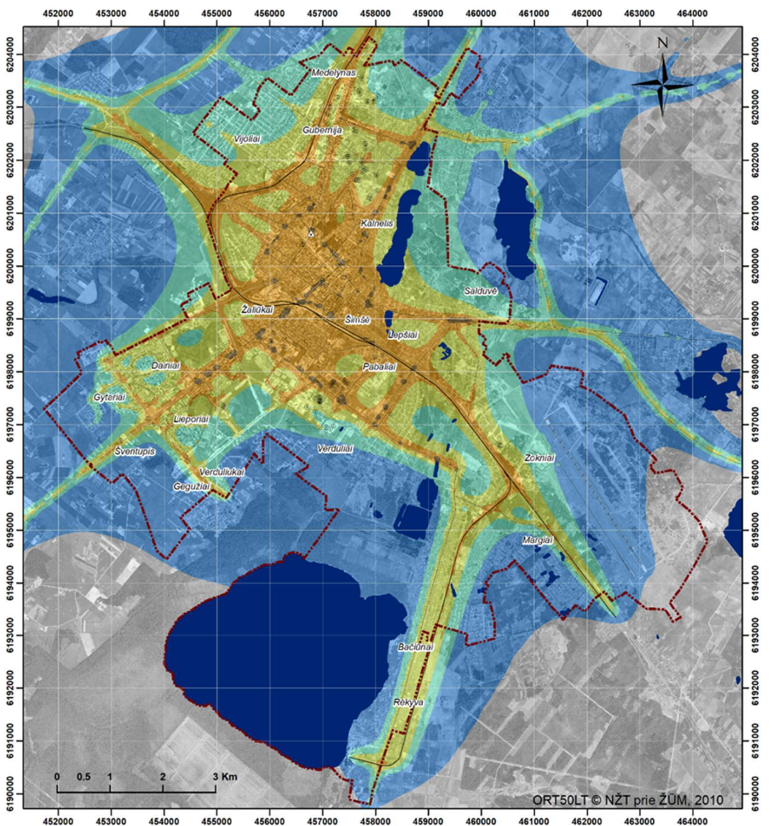
Vidutinė metinė azoto dioksido ( \text{NO}_2 ) koncentracija ( \mu\text{g}/\text{m}^3 ) aplinkos ore Šiauliuose 2019 m. Ribinė vertė 40 \mu\text{g}/\text{m}^3
