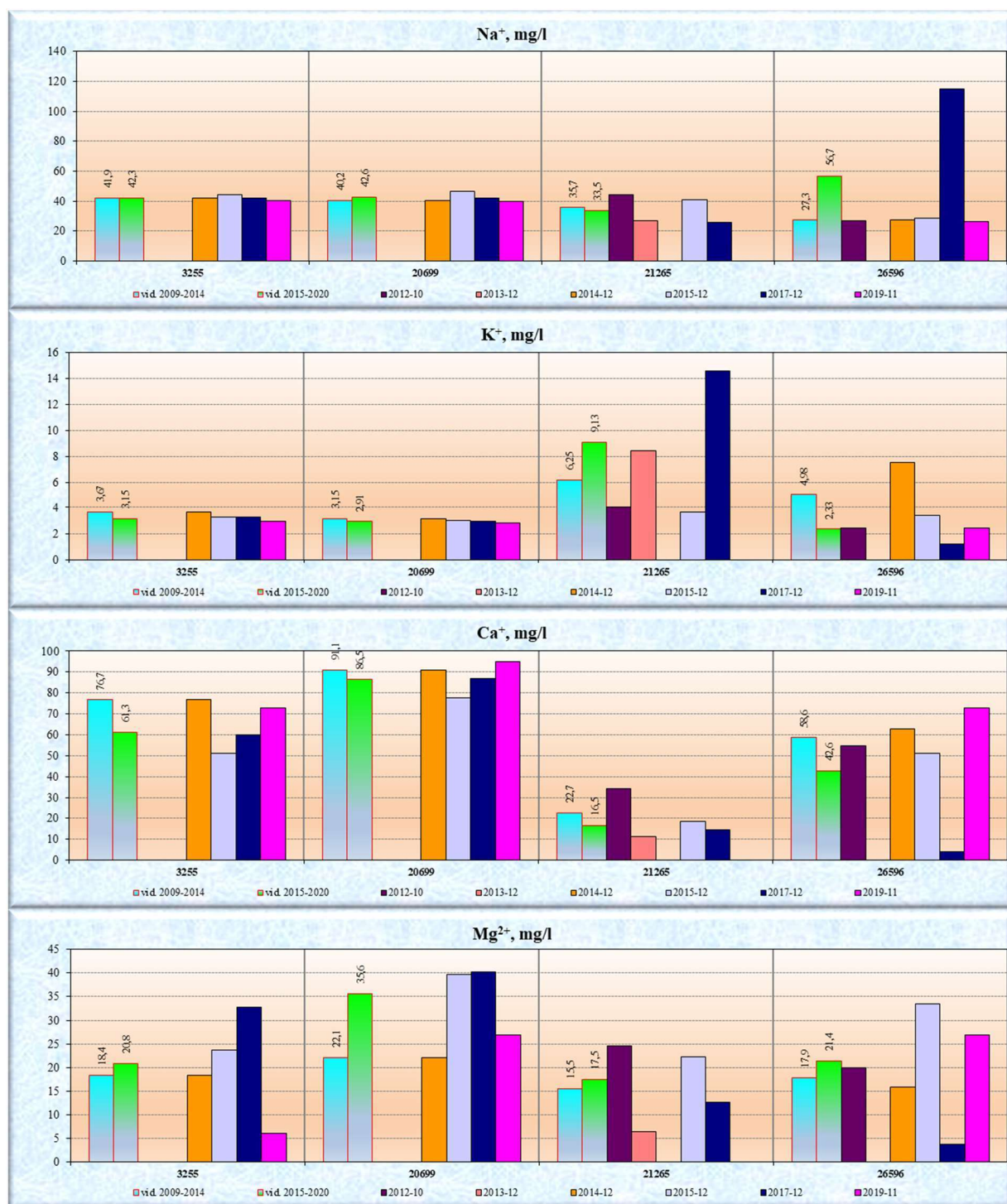
43 pav. Gręžinių viršutinio permo požeminio vandens cheminės sudėties pokyčiai 2012–2020 m. ir vidutinės koncentracijos (pagrindiniai anijonai)
