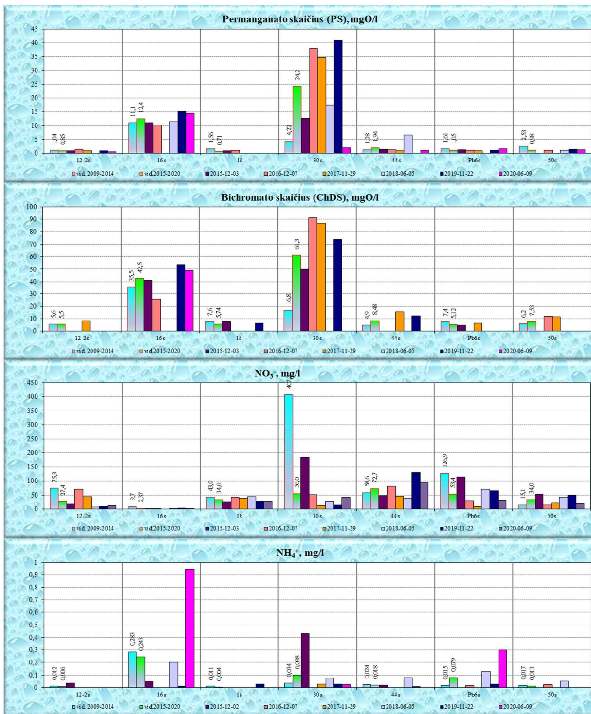
34 pav. Šulinių gruntinio vandens cheminės sudėties pokyčiai 2015–2020 m. ir vidutinės koncentracijos 2009–2014 m. (organinės medžiagos rodikliai, mineralinio azoto kiekis)
