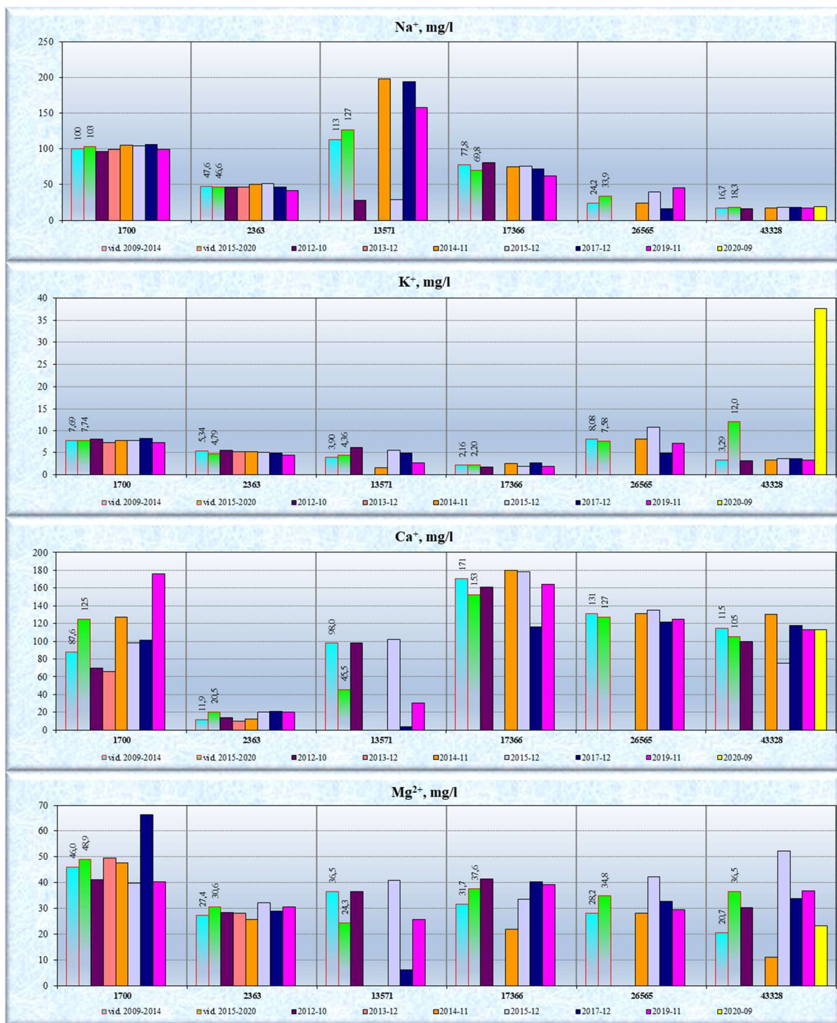
40 pav. Grėžinių tarpmoreninių sluoksnių vandens cheminės sudėties pokyčiai 2012–2020 m. ir vidutinės koncentracijos (pagrindiniai anijonai)
