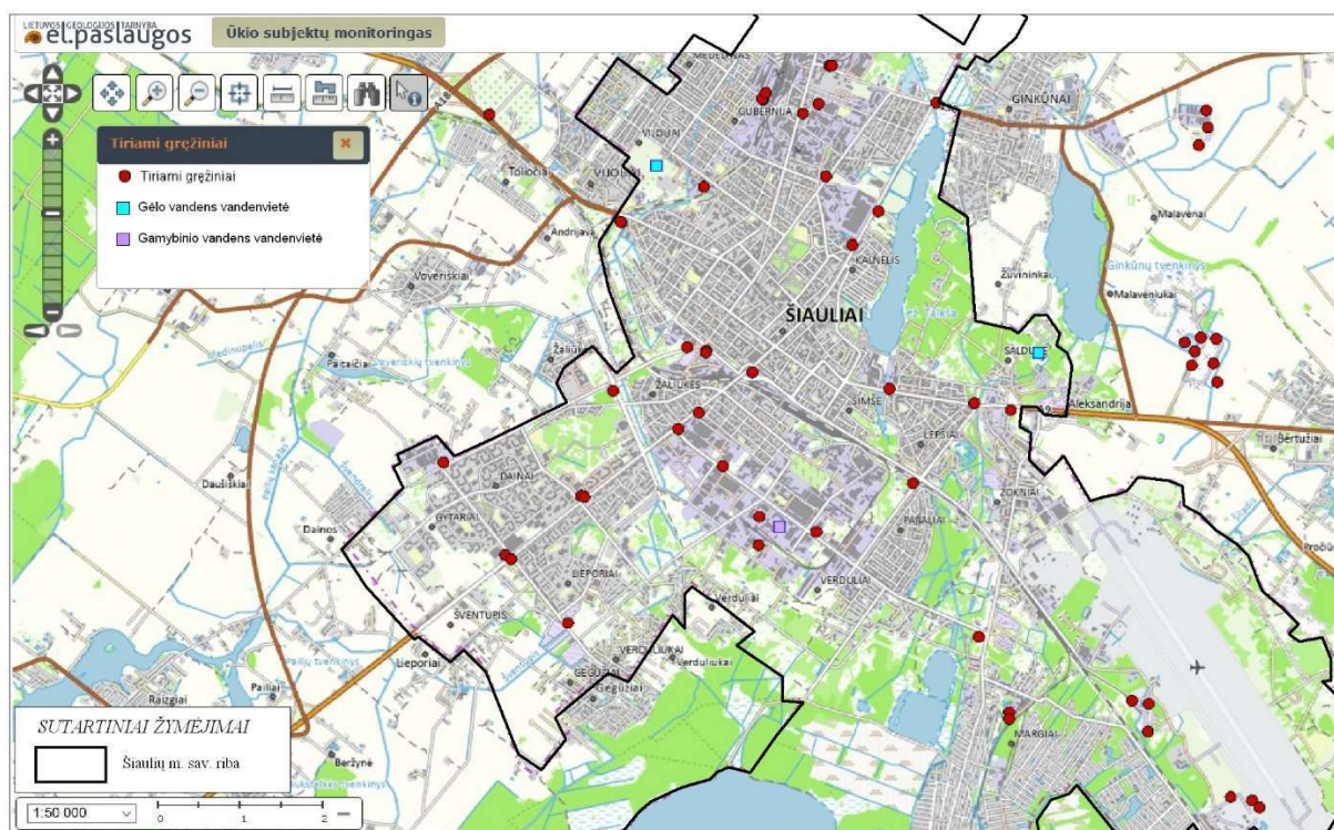
27 pav. Ūkio subjektų, vykdančių monitoringą, tiriamųjų gręžinių išdėstymo schema (pagal [16])
